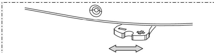
Détail commande de registre d'air primaire
