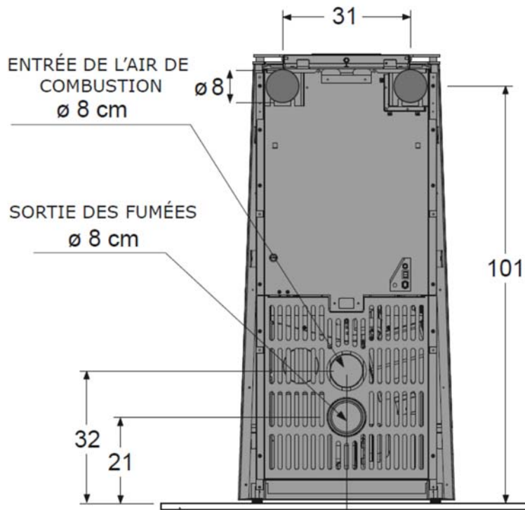
Figure 1 – Description d'un corps de chauffe ATLANTIS ou LXE
