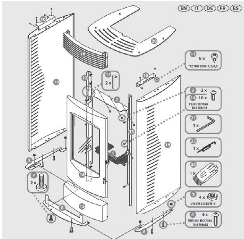
Figure 3 – Exemple de description d'un d'habillage "STEEL" pour corps de chauffe ATLANTIS ou LXE
